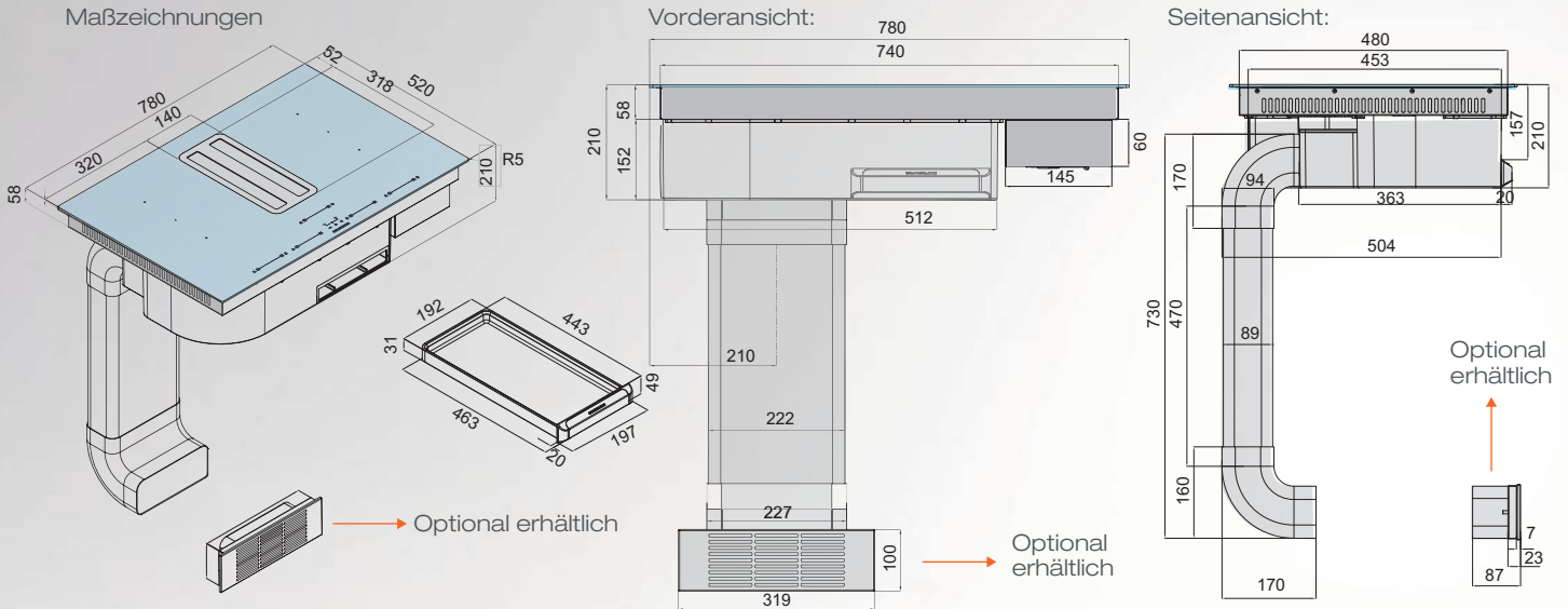
Maßzeichnungen
